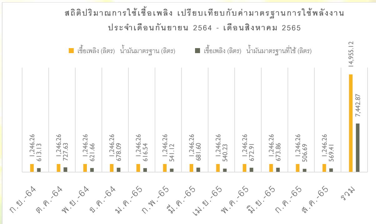
แผนภูมิ ๒ สถิติปริมาณการใช้เชื้อเพลิง เปรียบเทียบกับค่ามาตรฐานการใช้พลังงาน
